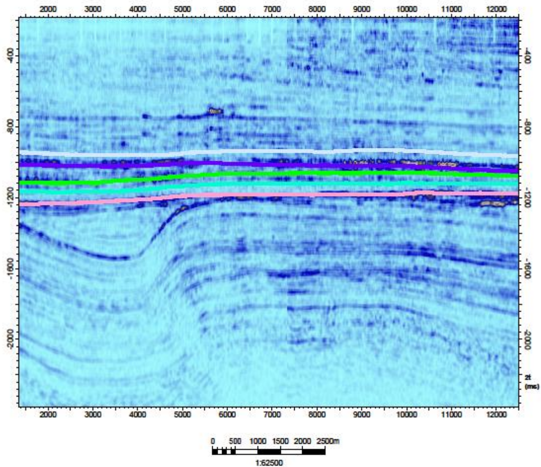
Legenda: — Pretpliocenska diskordancija — Santerno — PLQ-A — PLQ1-D — PLQ1-C Slika 5.5 Uzdužni profil 2100 prikazan atributom trenutne amplitude
