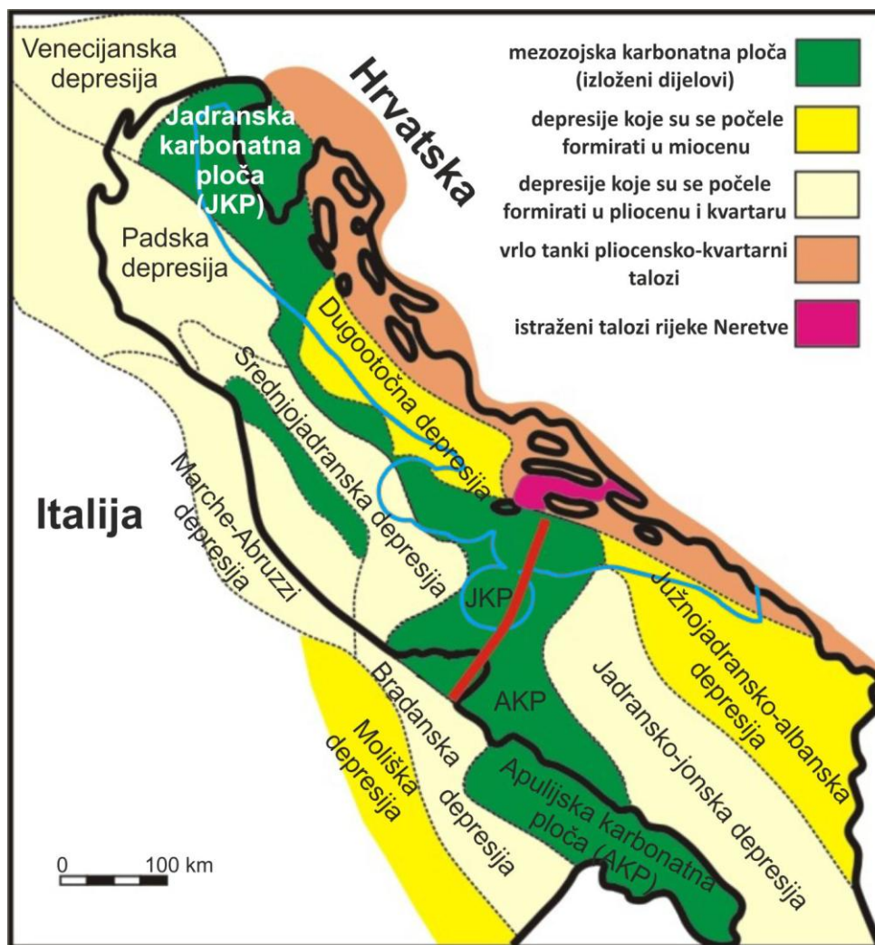
Slika 2.2 Miocenske i pliocensko-kvartarne depresije u Jadranskom bazenu (izmjenjeno prema Velić & Malvić, 2011; PRELOGOVIĆ & KRANJEC 1983)
