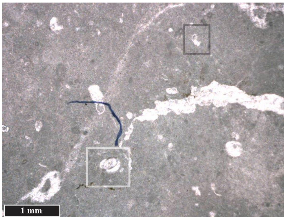
Slika 7-3. Mikrofotografija uzorka vapnenca TR-2. U mikritu su vidljive foraminifere iz porodice Discorbidae (tamno uokvireno područje) i foraminifere iz porodice Miliolidae (bijelo uokvireno područje).
