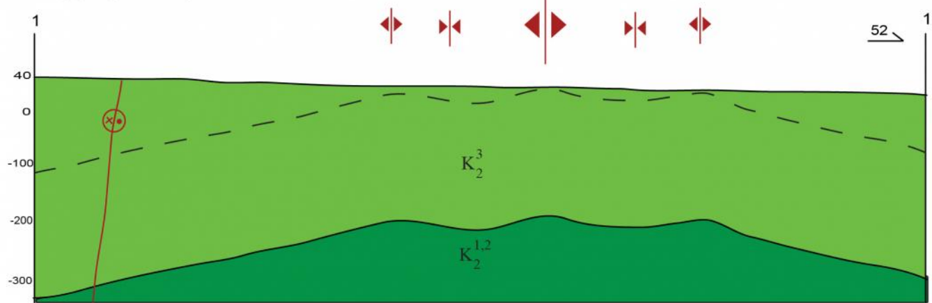
Profil 1 - 1' kroz vrh antiklinale (povećano mjerilo zbog preglednosti)
