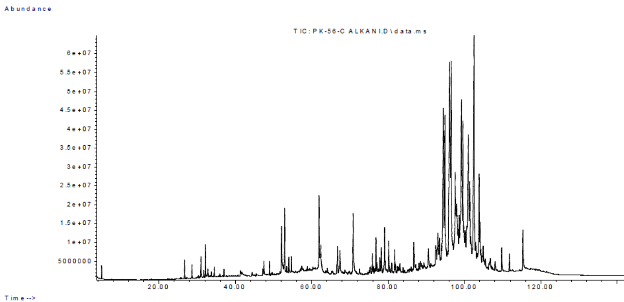
Slika 6.9: TIC kromatogram alkanske frakcije bitumena uzorka PK – 56C
