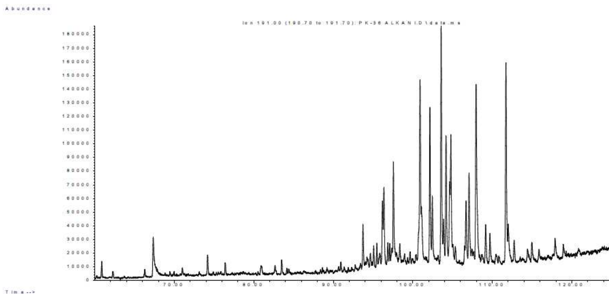
Slika 6.7: m/z 191 maseni kromatogram alkanske frakcije bitumena uzorka PK – 36
