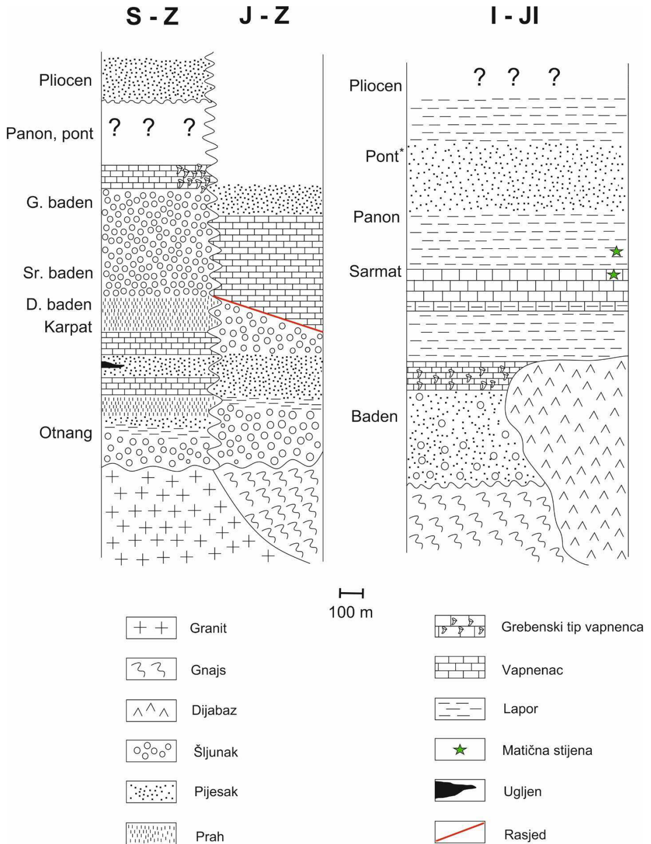
Slika 7.1: Geološki stupovi Požeške kotline
