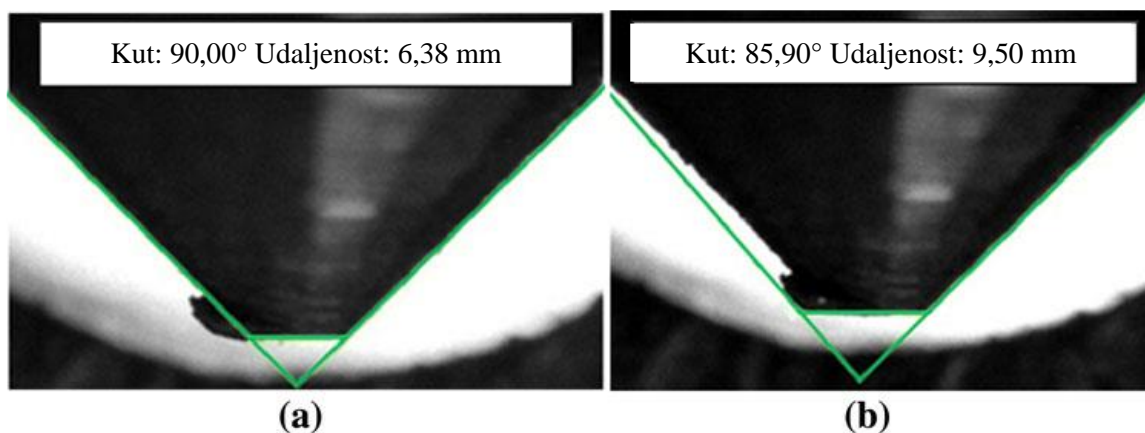
Slika 5-3. Prikaz mjerenja s bočnim prikazom na: (a) ispravan način i (b) neispravan način (Alber et al. 2013).
