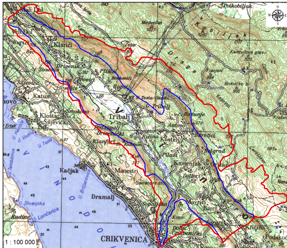
Slika 4-3. Kontura porječja rijeke Dubračine (crveni poligon) koje je geološki kartirano u mjerilu 1 : 25 000, a u sklopu koje se nalazi plavi poligon i predstavlja površinu koja je dodatno kartirana u mjerilu 1 : 5 000. Kartiranje je obavio Hrvatski geološki institut tijekom 2007. godine.
