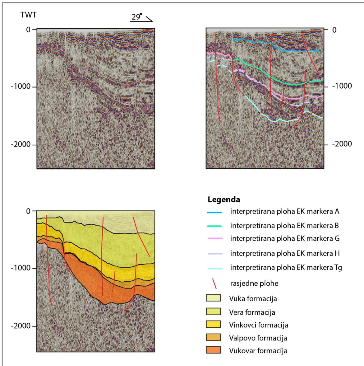
Slika 6.2. Dio interpretiranog seizmičkog profila A s vidljivo rasjedanom predneogenskom podlogom koju od mlađih naslaga odvaja horizont Tg; Zone omeđene ploham repernih horizonata predstavljaju izdvojene formacije iz jednostavnog modela – nema dislociranja horizonata po ploham rasjeda
