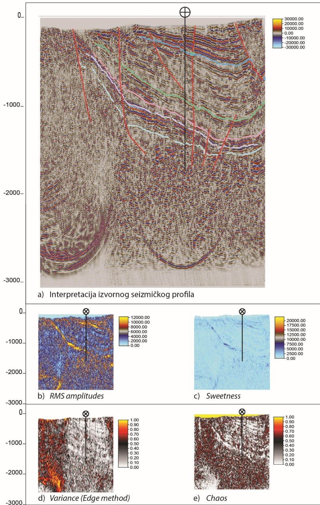
Slika 5.2. Primjeri nekoliko mogućih seizmičkih atributa prikazanih na seizmičkom profilu B iz Požeške kotline (modificirano prema Brcković et al., 2017)
