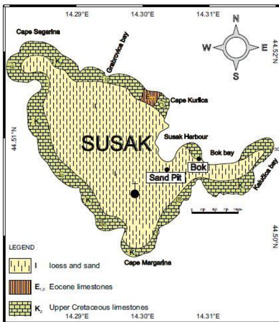
Slika 2.2. Pojednostavljena geološka karta otoka Suska.
