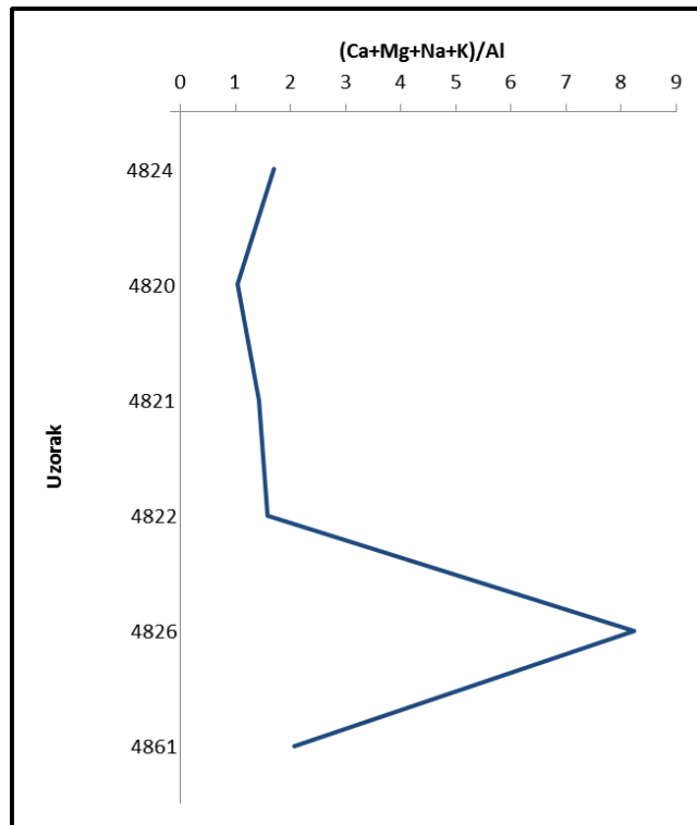
Slika 4.2. Omjer \Sigma(\text{Ca}, \text{Mg}, \text{Na}, \text{K})/\text{Al} . Uzorci su poredani po dubini.
