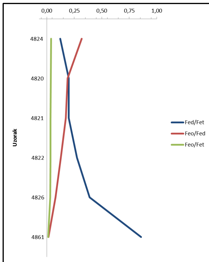
Slika 4.18. Omjeri \text{Fe}_d/\text{Fe}_t , \text{Fe}_o/\text{Fe}_d i \text{Fe}_o/\text{Fe}_t .
