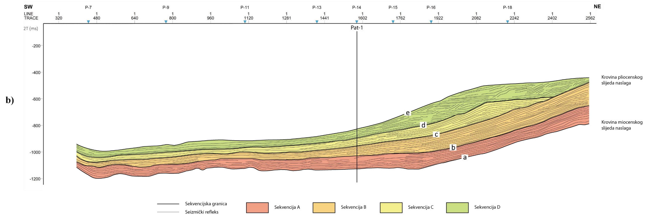
Slika 5-3: Odabrani referentni seizmički profil AB (a) s odgovarajućom interpretacijom (b).
