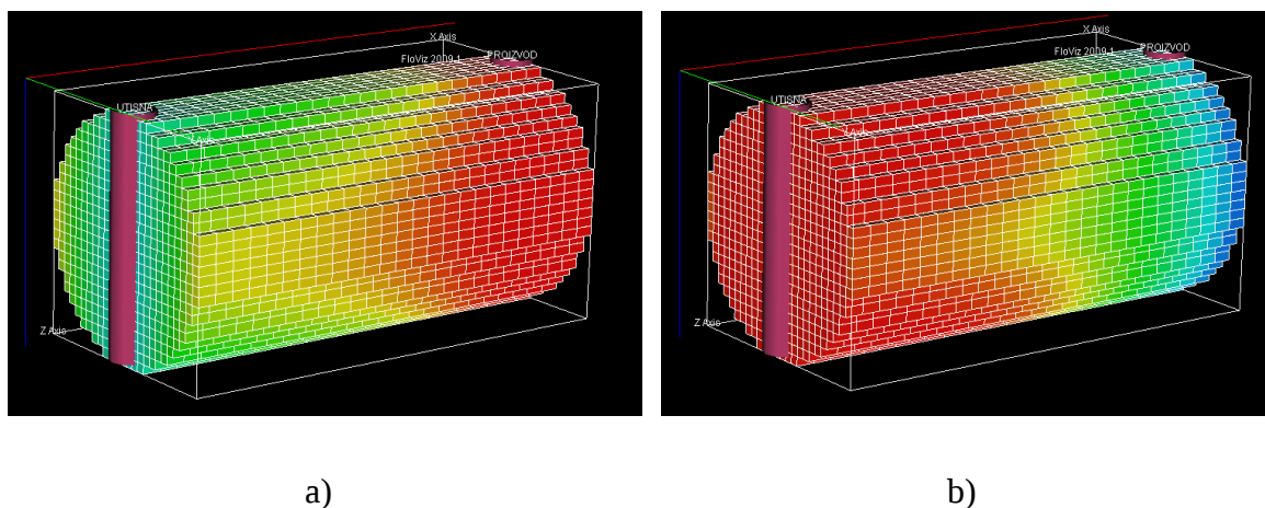
Slika 5-6. Vizualizacija rezultata simulacije: a) Promjena zasićenja ulja u jezgri; b) Promjena koncentracije polimera u jezgri
