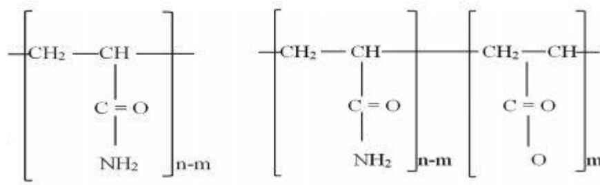
Slika 2-3. Struktura poliakrilamida (PAM) i djelomično hidroliziranog poliakrilamida (HPAM) (Romero-Zeron, 2016)
