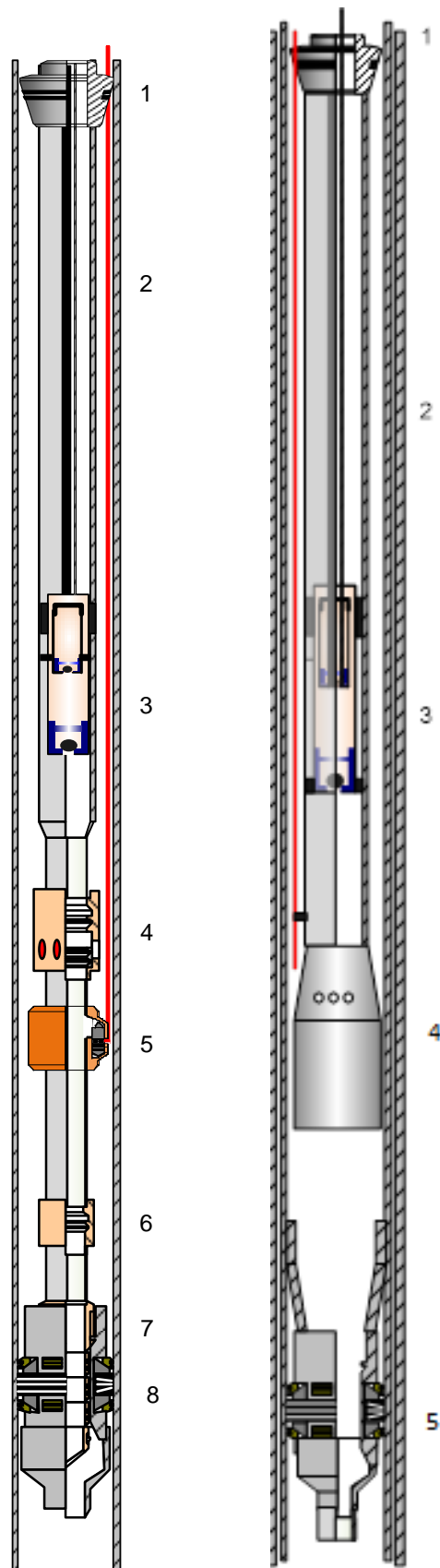
Slika 5-2. Tipična oprema u području od proizvodnog pakera do ušća s hermetičnom (lijevo) i nehermetičnom (desno) postojećom eksploatacijskom kolonom zaštitnih cijevi (INA d.d., 2017 b)
