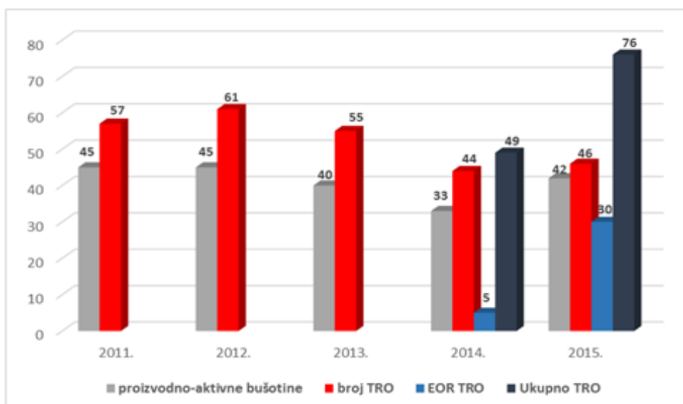
Slika 3-1. Broj tekućih remonata opreme (TRO) u odnosu na broj proizvodnih bušotina po godinama (INA d.d., 2017 b)
