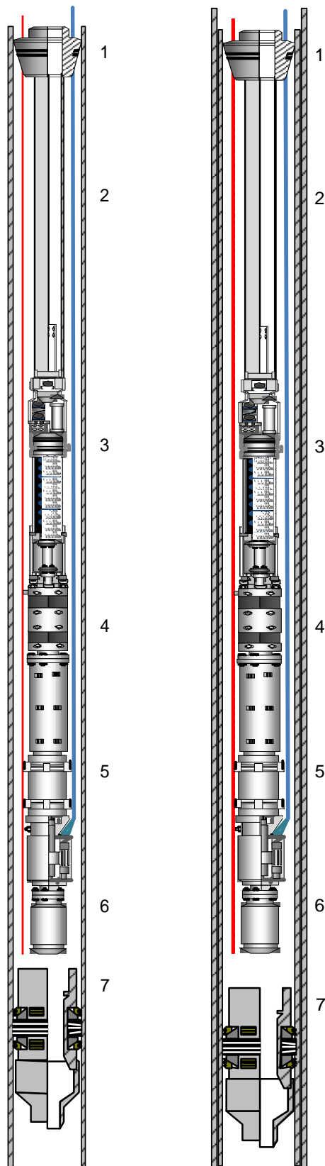
Slika 5-3. Tipaska oprema u području od proizvodnog paker do ušća s hermetičnom (lijevo) i nehermetičnom (desno) postojećom eksploatacijskom kolonom zaštitnih cijevi za bušotine s centrifugalnom sisaljkom (INA d.d., 2017 b)
