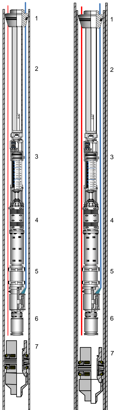
Slika 5-3. Tipska oprema u području od proizvodnog paker do ušća s hermetičnom (lijevo) i nehermetičnom (desno) postojećom eksploatacijskom kolonom zaštitnih cijevi za bušotine s centrifugalnom sisaljkom (INA d.d., 2017 b)
