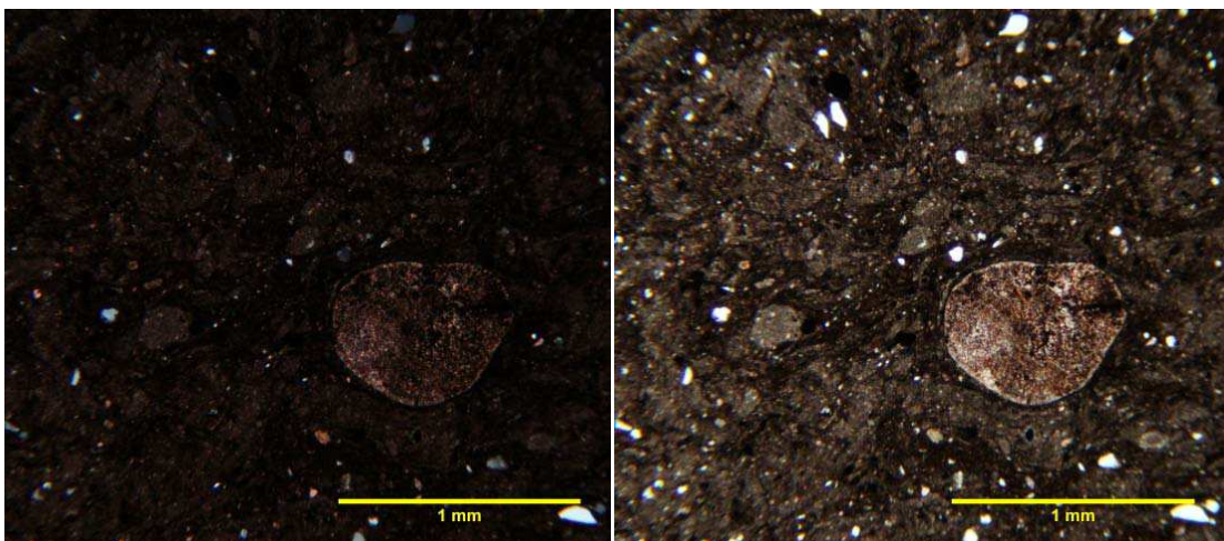
Slika 4.46. Mikrofotografije uzorka Bruvno 3a, s analizatorom (a) i bez analizatora (b). Litična grauvara.
