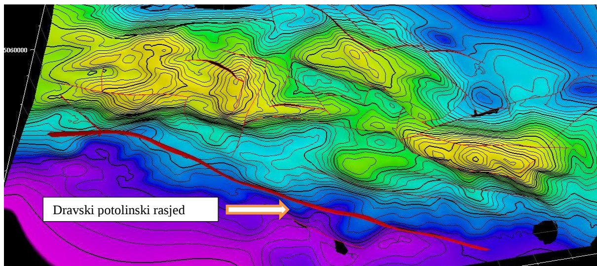
Slika 7-2. Strukturalna karta po plohi repera Tg; strelicom je označen glavni Dravski potolinski rasjed koji se pruža duž sjevernog ruba Đakovačko – vinkovačkog ravnjaka.
