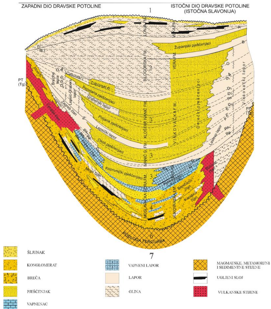
Slika 4-1. Shematski litostratigrafski presjek neogensko-kvartarnog kompleksa u stupovima dubokih bušotina na području Dravske potoline ( www.azu.hr , modificirano prema ŠIMON, 1980 ).
