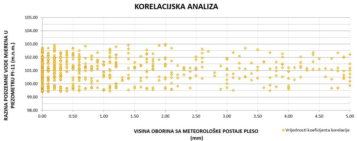
Slika 6-2. Ponovljena korelacijska analiza (maksimalna korelacija) za vodocrpilište Velika Gorica i meteorološku postaju Pleso
