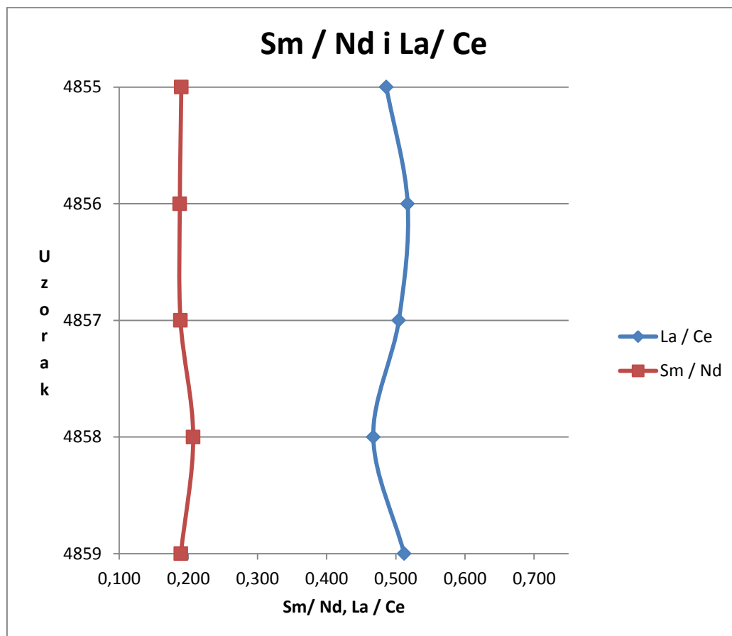
Slika 5.10. Omjeri Sm/Nd i La/Ce
