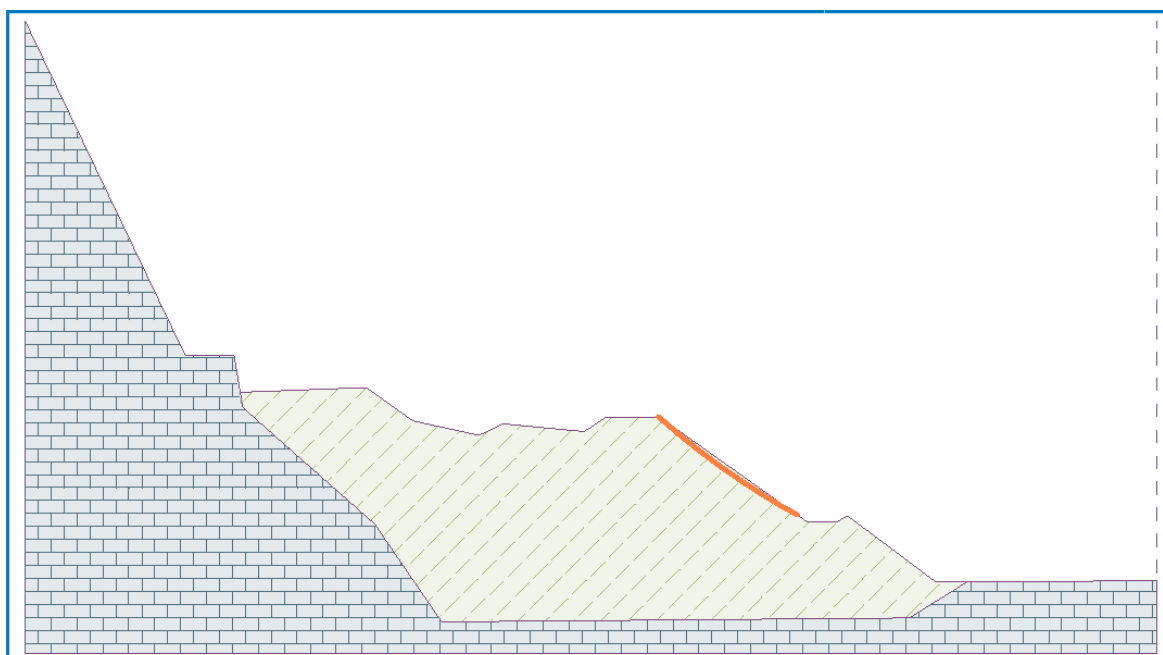
Slika 4-7. Klizna ploha za vrijednosti c_{ef} = 0,1 kPa, \varphi_{ef} = 36^\circ i F_s = 1,05 u profilu 6
