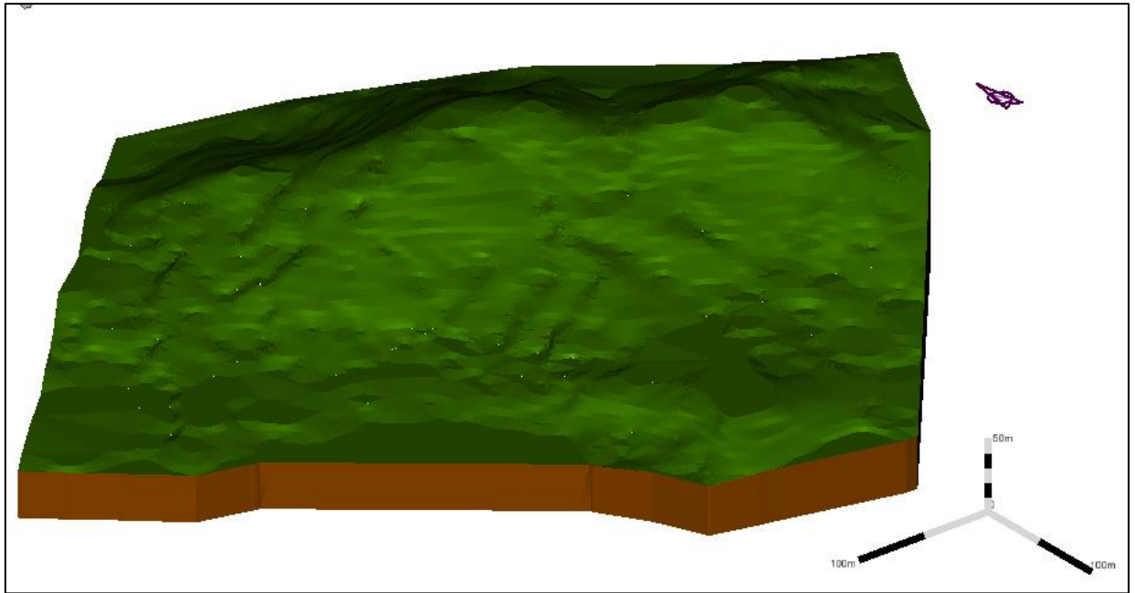
Slika 4-7. Triangulirani 3D model šireg područja Istražnog prostora „Vrebač“
