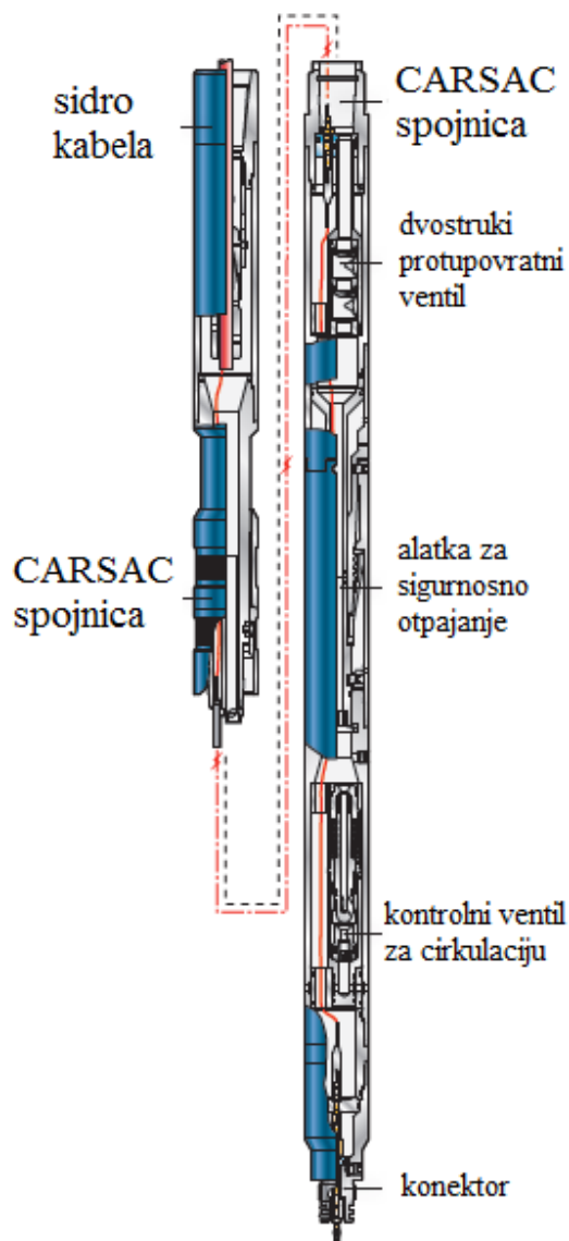
Slika 5-25. Dubinski sklop alatke savitljivog tubinga za provođenje karotažnih ispitivanja tvrtke NOV Coiled Tubing Tools (National Oilwell Varco, 2016)
