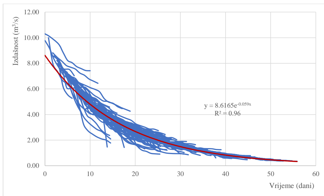
Slika 3.6. Glavna recesijska krivulja za izvor Gradole
