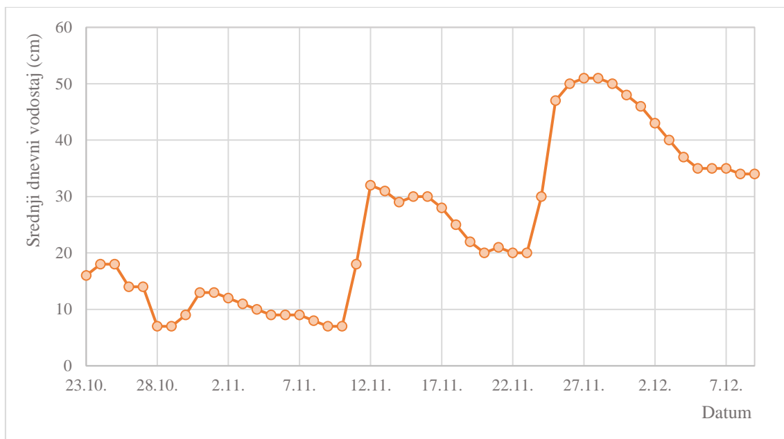
Slika 3.7. Promjena vodostaja u vremenu na izvoru Gradole
