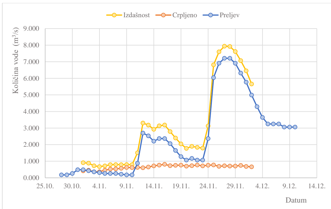
Slika 3.8. Prikaz količine vode na preljevu izvora, crpljene količine te kao zbroj, ukupne izdašnosti izvora
