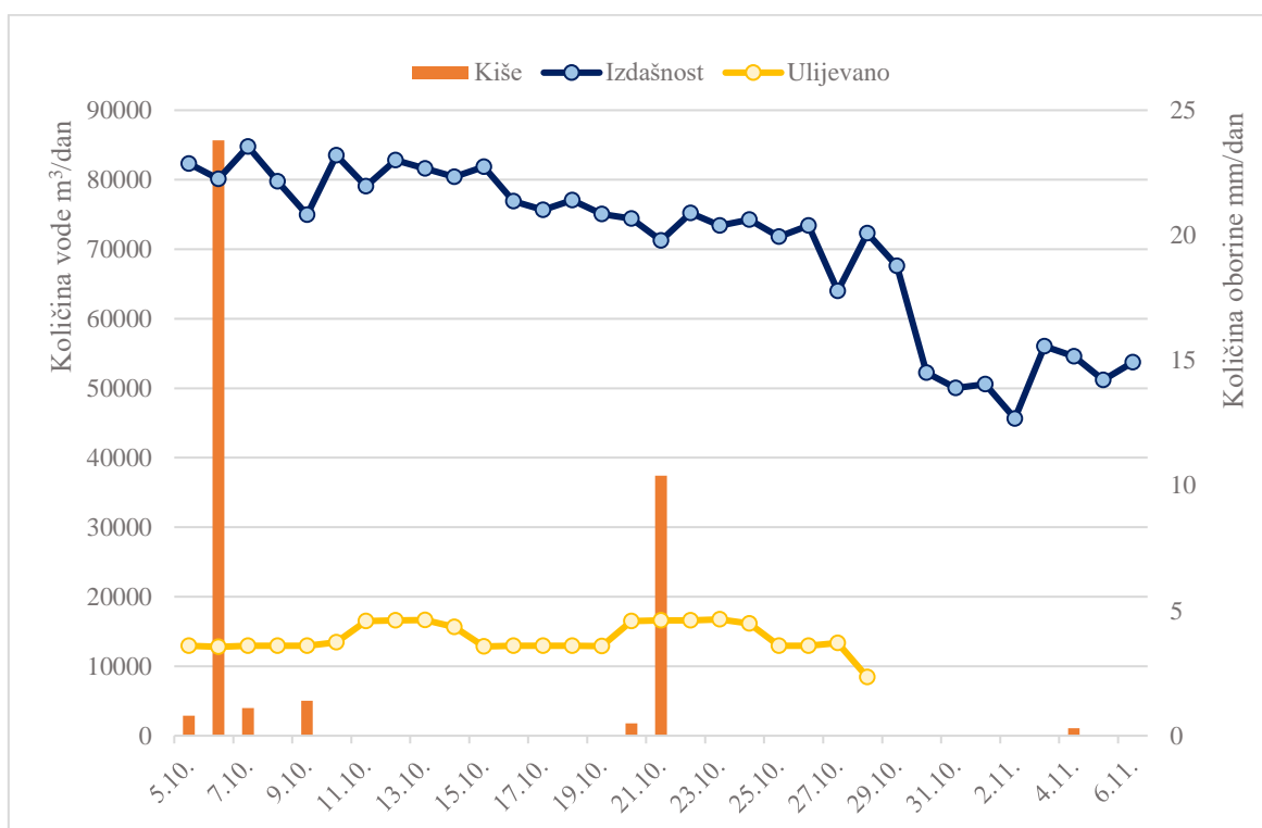
Slika 5.4. Prikaz izdašnosti izvora, ulijevane vode i kišnih epizoda od 5.10. do 7.11.
