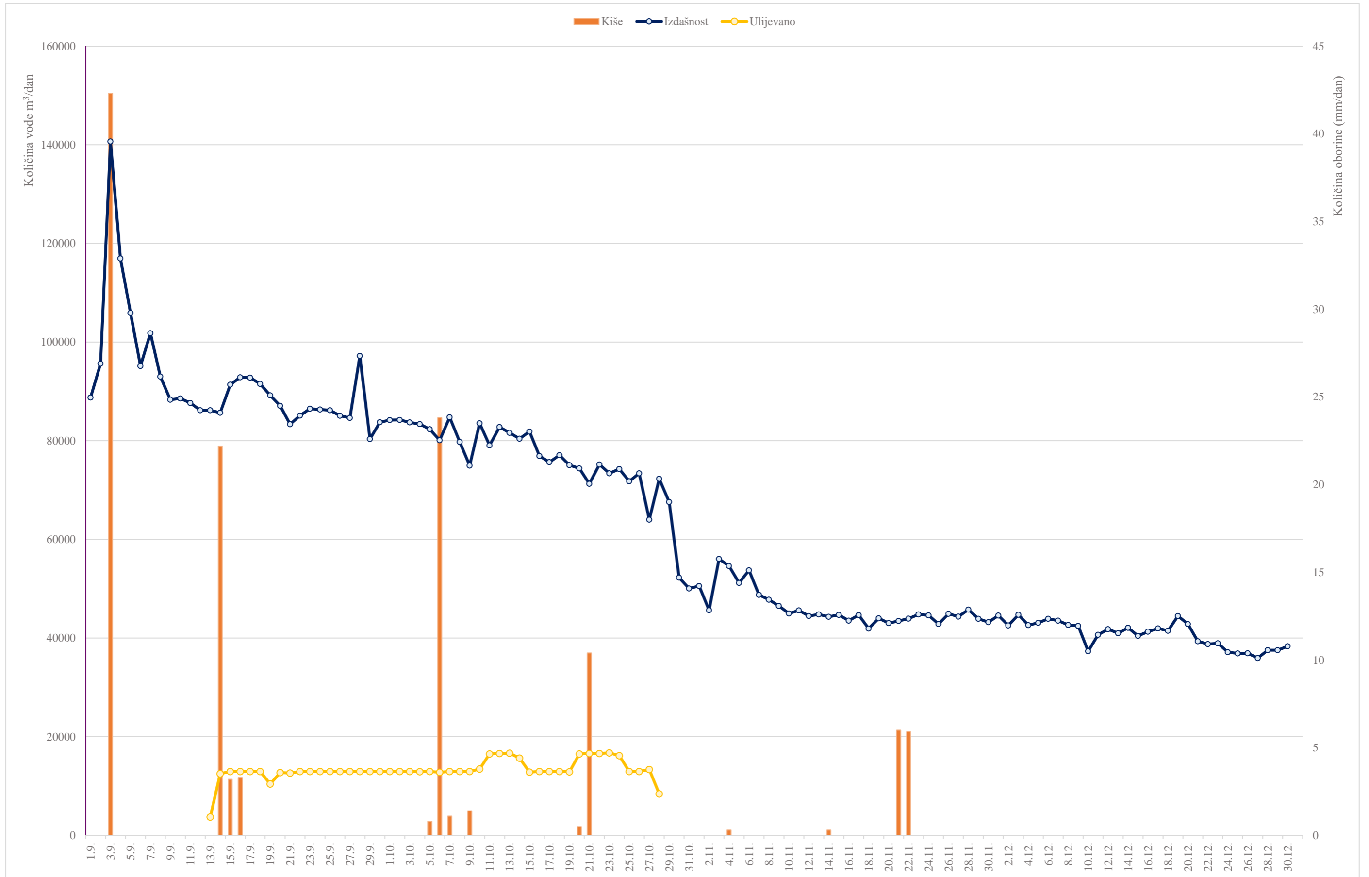
Prilog 1. Prikaz izdašnosti izvora ( \text{m}^3/\text{dan} ), uz količinu ulijevane vode u ponor ( \text{m}^3/\text{dan} ) te kiše u promatranom razdoblju ( \text{mm}/\text{dan} )
