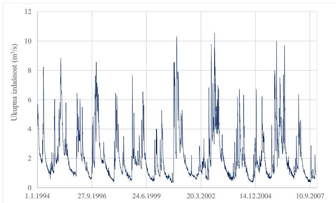
Slika 3.5. Dnevni protoci izvora Gradole u razdoblju od 1.1.1994. do 31.12.2007.
