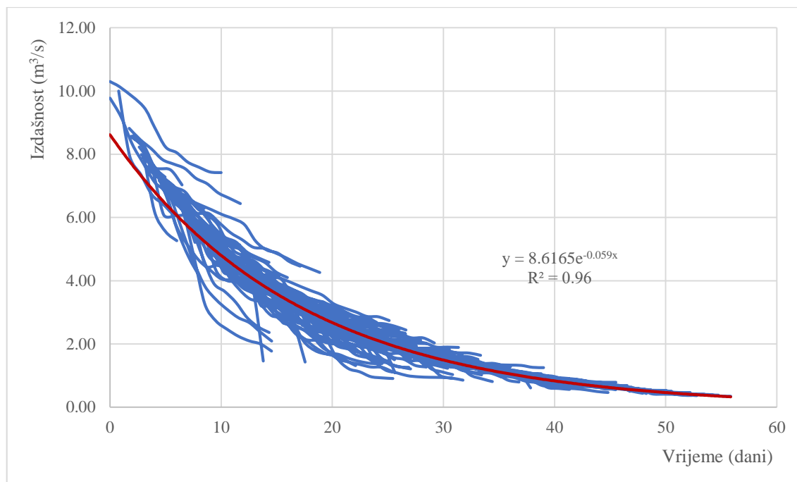
Slika 3.6. Glavna recesijska krivulja za izvor Gradole
