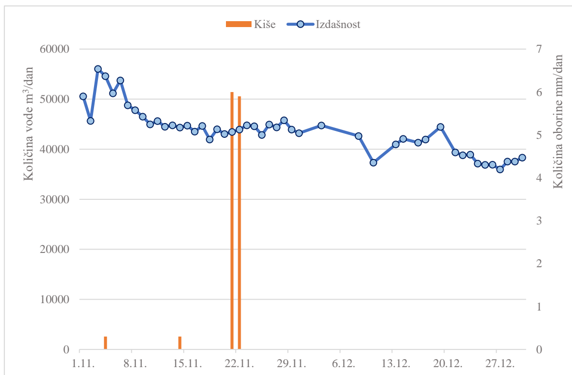
Slika 5.5. Prikaz izdašnosti izvora, ulijevane vode i kišnih epizoda od 1.11. do 31.12.
