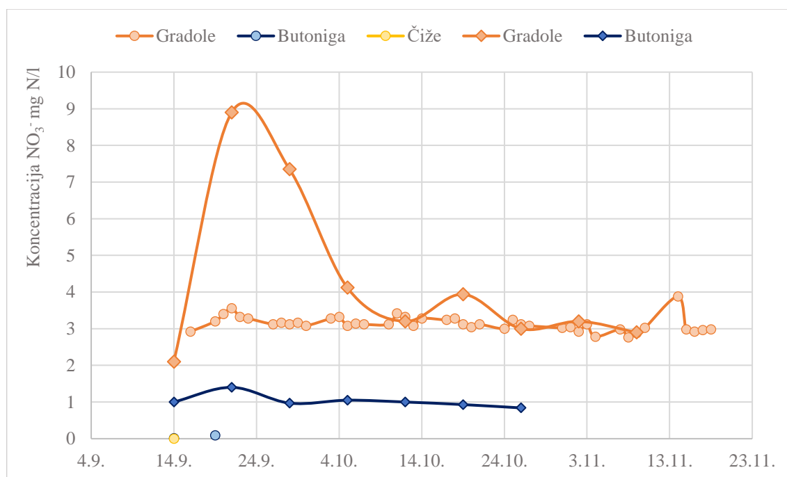
Slika 4.4. Koncentracija nitrata na izvoru Gradole (mjerena svakodnevno i tjedno), vodi ulijevanoj u ponor te u akumulaciji Butoniga (svakodnevno i tjedno).
