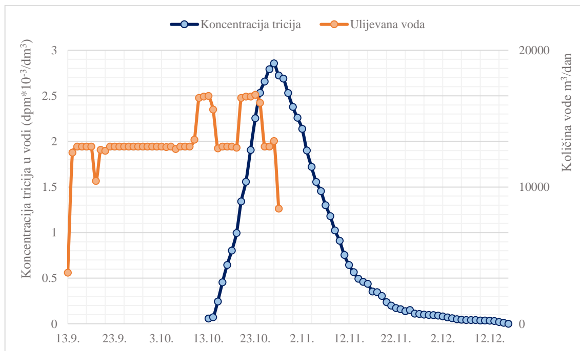
Slika 5.1. Prikaz koncentracije tricija u uzorcima vode o vremenu proteklom od trasiranja i količine ulijevane vode u ponor Čiže
