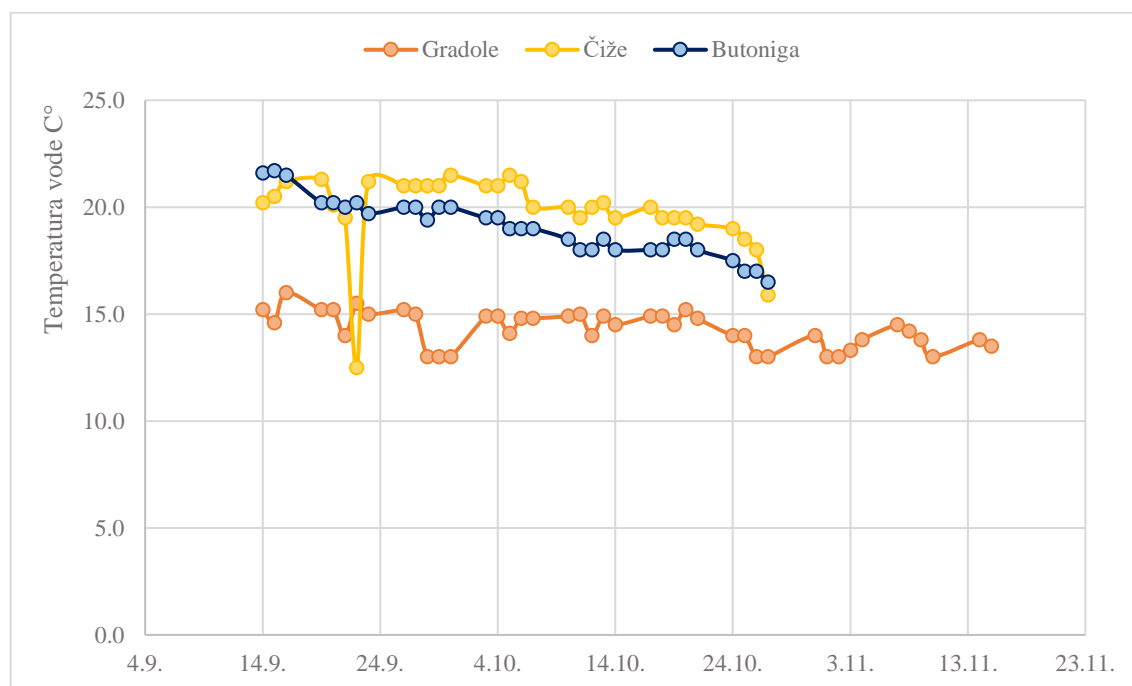
Slika 4.3. Temperatura vode mjerena na izvoru Gradole, ponoru Čiže i akumulaciji Butoniga.
