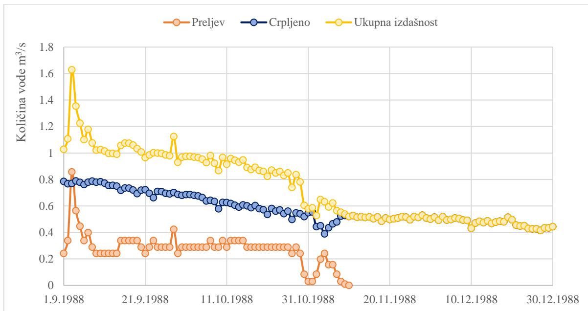
Slika 4.1. Prikaz količine vode na preljevu, crpne količine, te ukupne izdašnosti za izvor Gradole od 1.9. do 31.12.1988. godine
