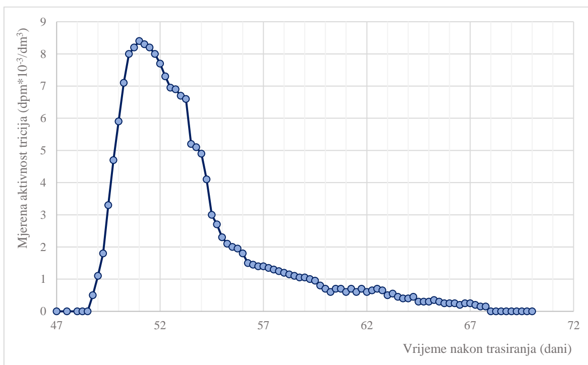
Slika 3.9. Mjerenja aktivnosti tricija u odnosu na vrijeme proteklo od trasiranja
