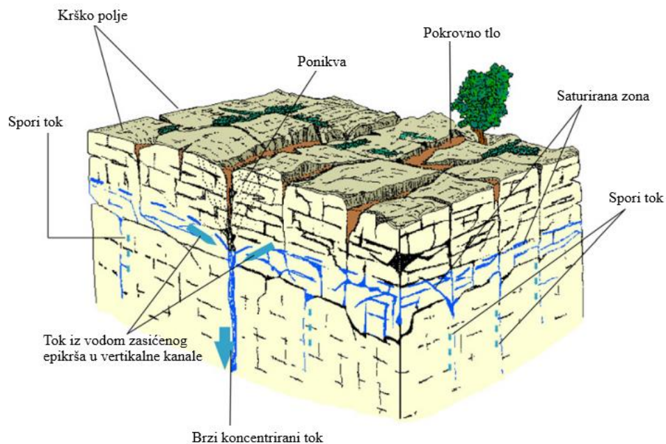
Slika 2.1. Prikaz epikrša, zadržavanja vode u saturiranoj zoni i podjele tokova na spori i brzi ulaskom u vadoznu zonu (prema Bakalowicz, 2005).
