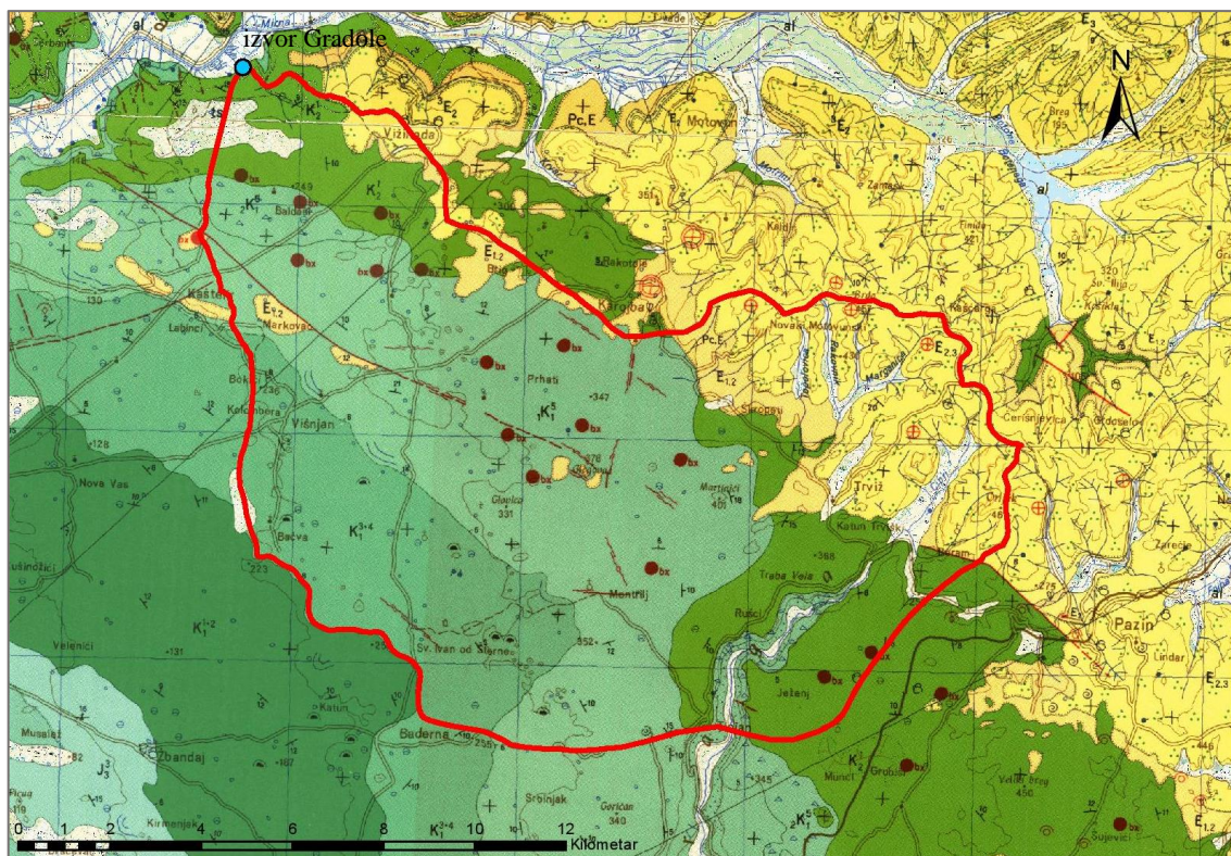
Slika 3.3. Geološka karta sliva izvora Gradole (OGK 1: 100 000, listovi Rovinj (Polšak i Šikić, 1969) i Trst (Anonimno, 1951-1964)). Kartirane jedinice: donja kreda (Barem - Apt K_1^{3+4} , Alb 1K_1^5 ), gornja kreda (Cenoman K_2^1 ), paleogen (Miliolidni vapnenac Pc, E 1 , Alveolinski i numulitni vapnenac E 1,2 , Flišne naslage E 2,3 ), kvartar q (terra rossa ts, aluvijani nanos al).
