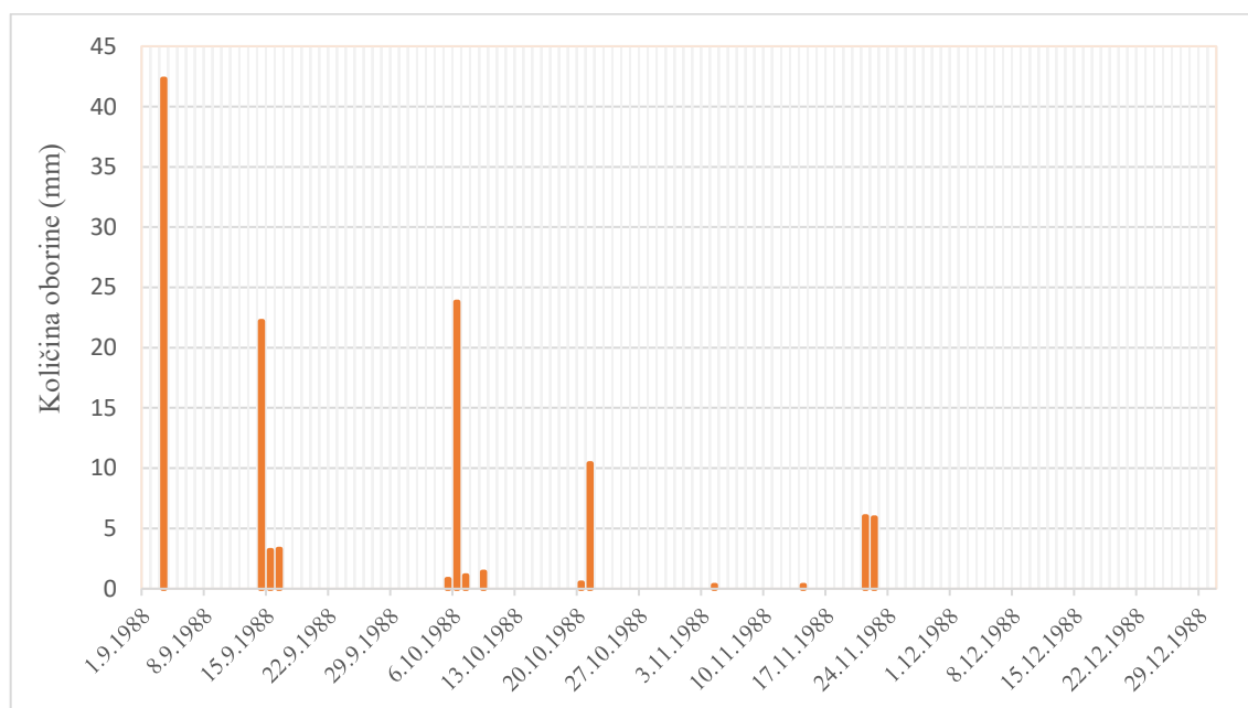
Slika 4.2. Dnevne oborine u razdoblju od 1.9. do 31.12.1988 godine
