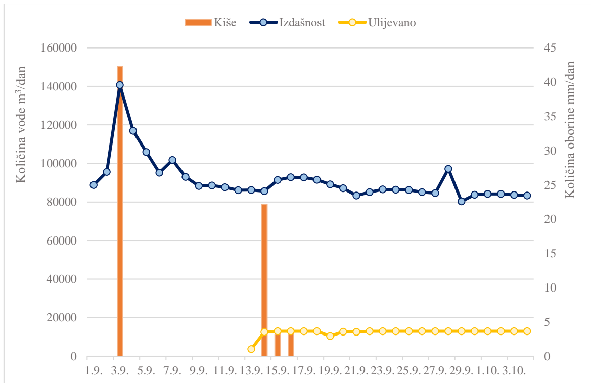
Slika 5.3. Prikaz izdašnosti izvora, ulijevane vode i kišnih epizoda od 1.9. do 4.10.
