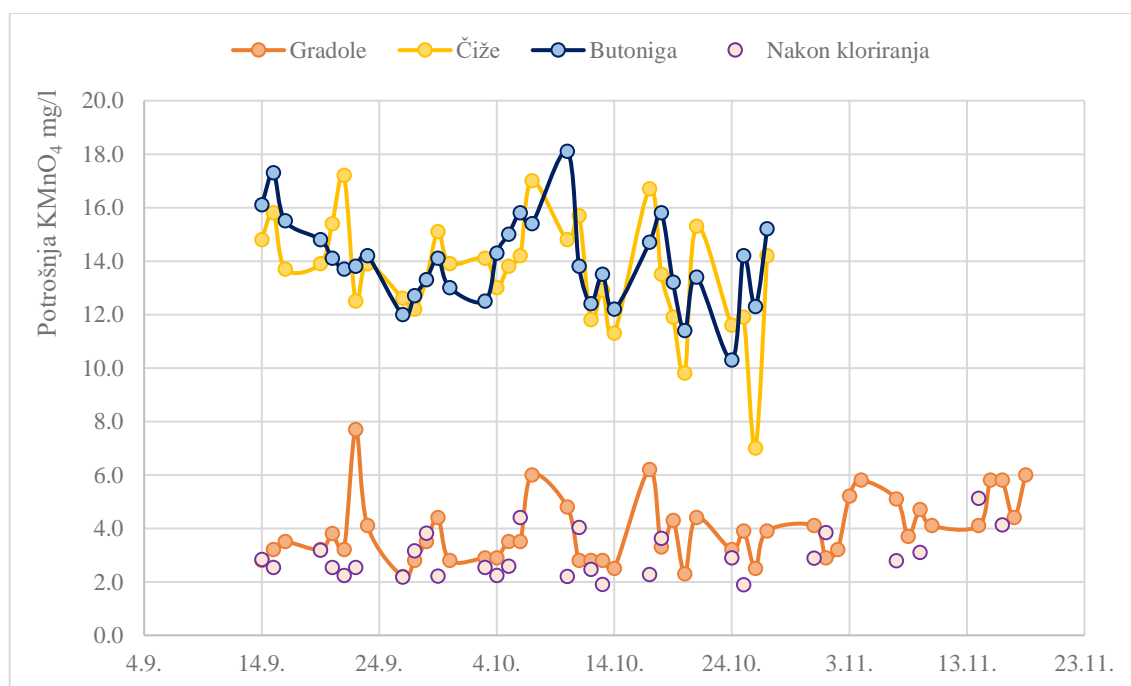
Slika 4.5. Utrošak kalij permanganata na izvoru Gradole (prije i nakon kloriranja), vodi ulijevanoj u ponor, vodi iz akumulacije Butoniga.
