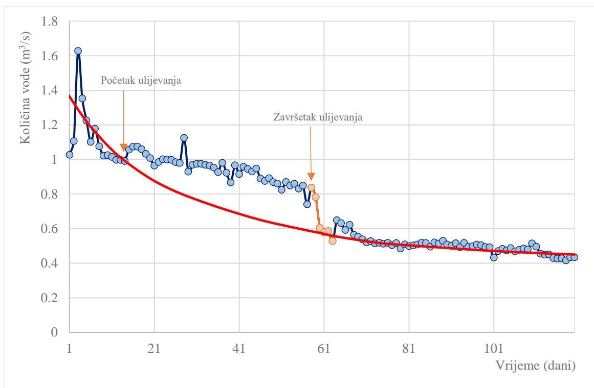
Slika 5.2. Prikaz promjene izdašnosti izvora Gradole u vremenu te aproksimirane glavne recesijske krivulje za promatrano razdoblje.
