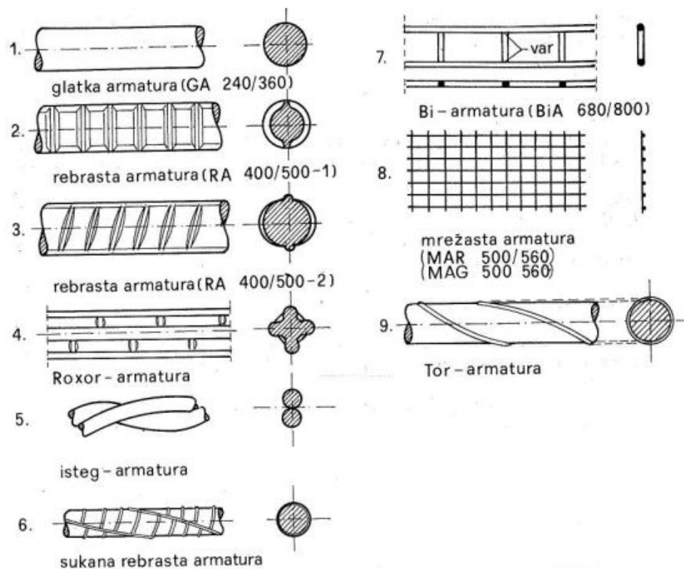
Slika 4-2. Različiti oblici čelične armature (Gukov, 2017)
