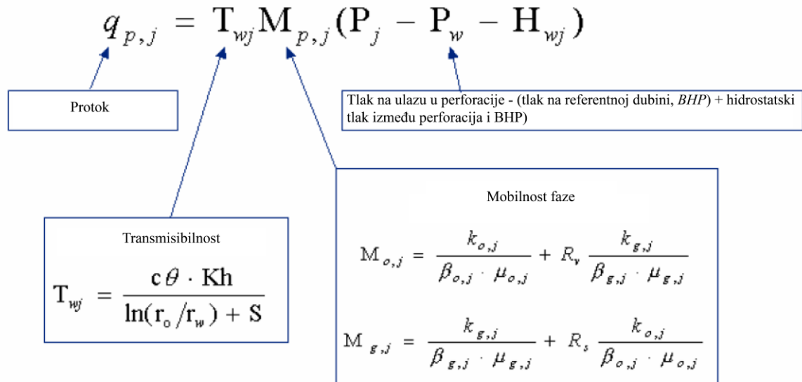
Slika 2-8. Set jednačbi za model bušotine (Schlumberger, 2015)
