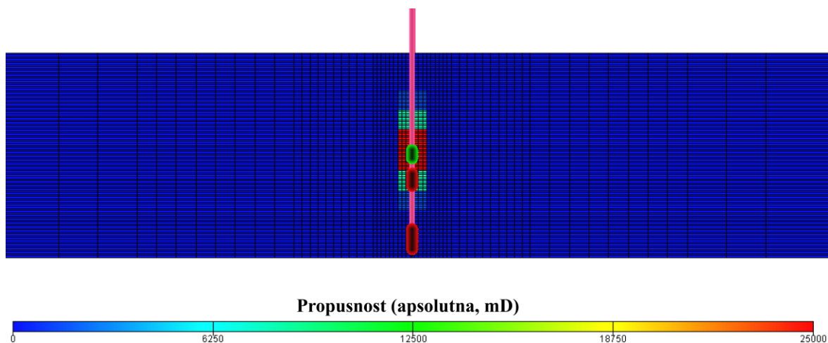
Slika 4-7. Model frakture x_f=3,5m , w_f=6,5mm , h_f=40m u softveru „Eclipse“
