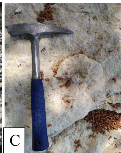
Slika 5-5. Moguće slampiranje u peloidnom grejnstonu (A, točka opažanja K-56), nodularna grada kalciferskog vapnenca (B, točka opažanja K-83) i detalj površine amonita (C, kamp Kašeja, južno od Medulina).
