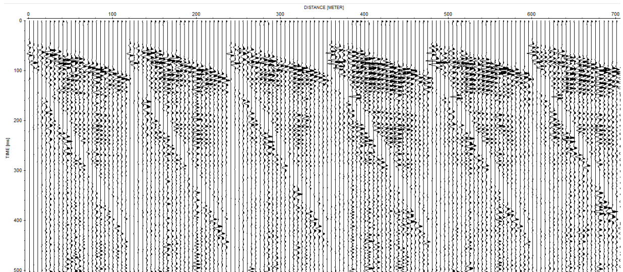
Slika 5-6 Isječak filtriranog profila nakon provedenog automatskog podešavanja amplituda.
