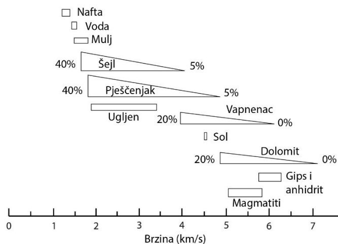
Slika 3-3 Brzine primarnih valova za različite litologije. Graf za šejl, pješčenjak, vapnenac i dolomit prikazuje također i ovisnost o poroznosti (izražena u postotcima). (Press, 1966; Gardner i dr., 1974 i Lindseth, 1972)
