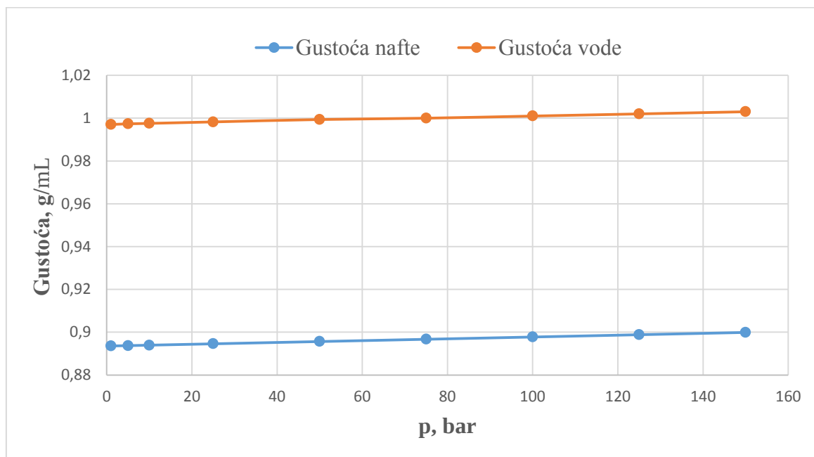
Slika 5-4. Promjena gustoće sirove nafte i vode s porastom tlaka
