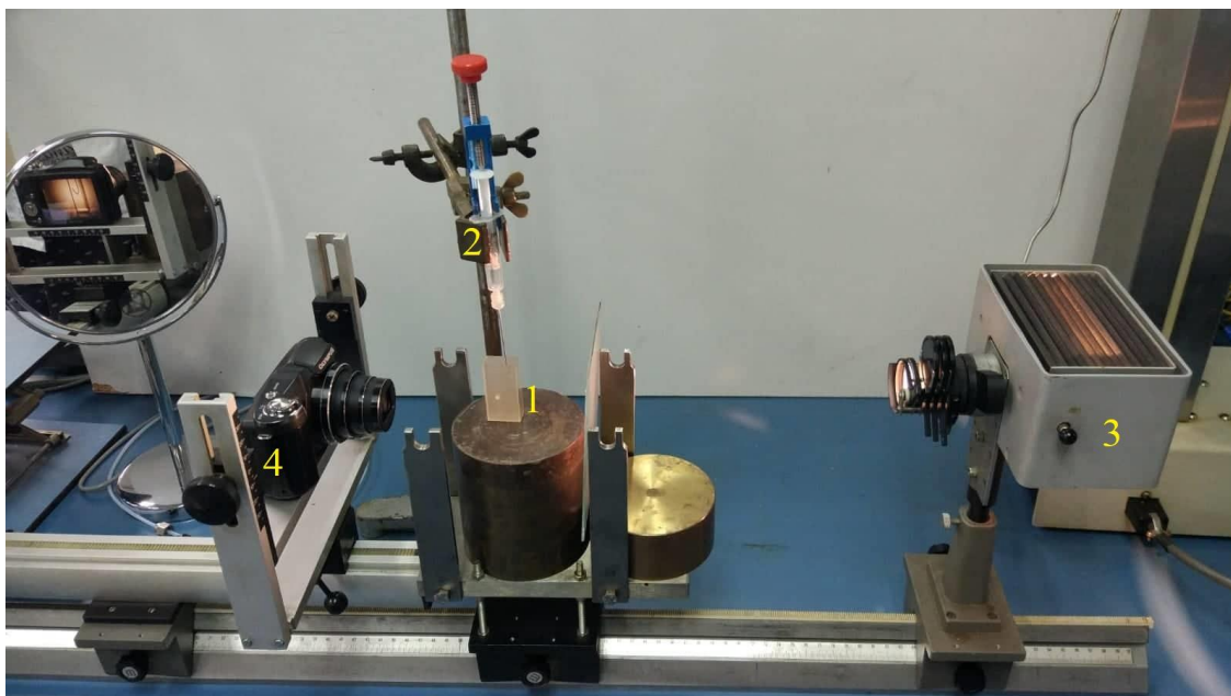
Slika 3-1. Prikaz aparature za mjerenje pri uvjetima sobne temperature i atmosferskog tlaka:
