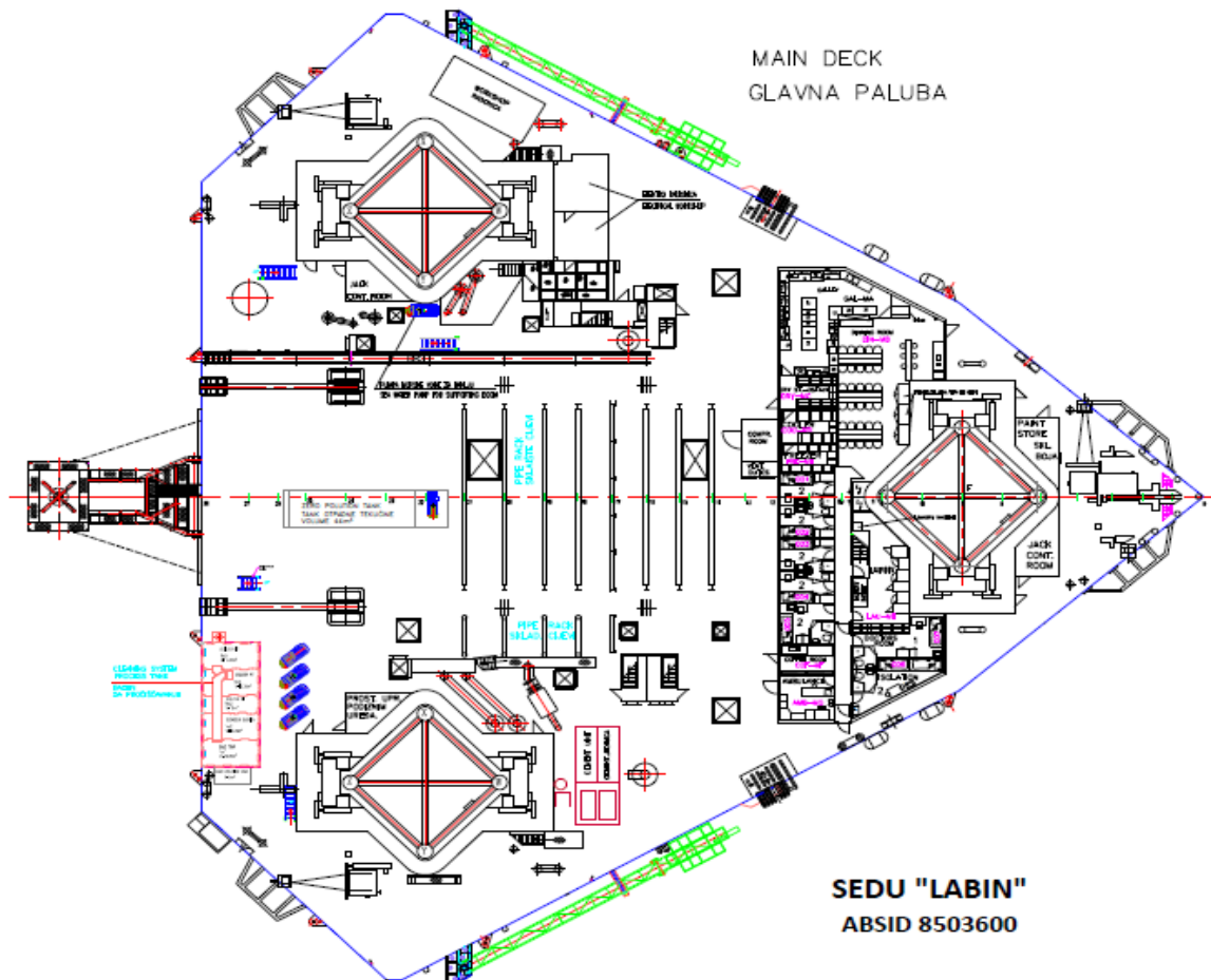
Slika 3-2. Tlocrt glavne palube platforme Labin (Izvešće tvrtke Adriatic Sub d.o.o. – Croscio, 2012)
