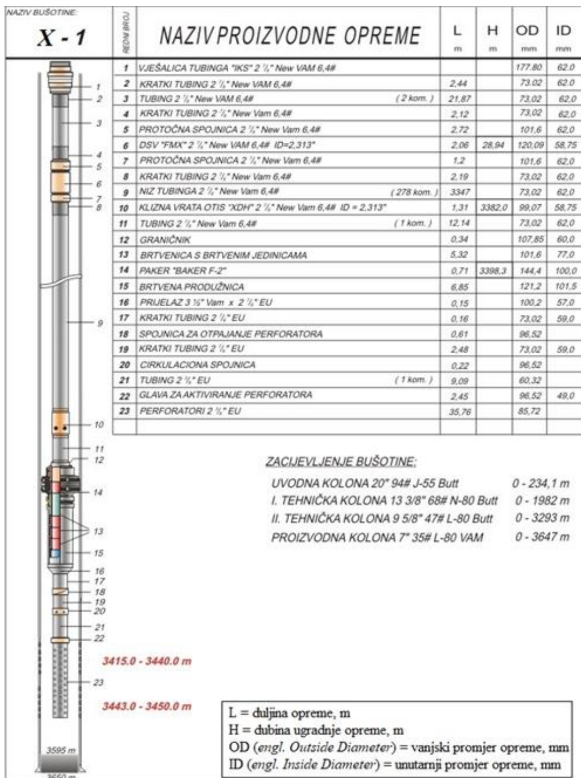
Slika 4-1. Početno proizvodno opremanje bušotine X-1 od 1989. do 2016. godine (Tehnička dokumentacija INA d.d., 2009)
