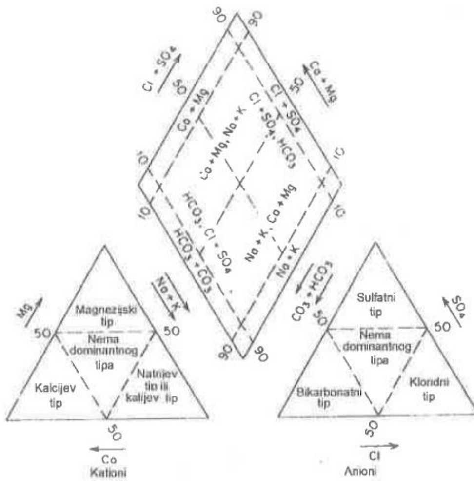
Slika 3.2. Prikaz vodnih facijesa u Piperovu dijagramu (Freeze, 1979; Halle, 2004)
