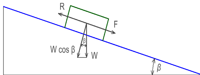
Slika 3-3 Mehanizam klizanja niz kosinu (Bošković i Šimunović, 2013)
