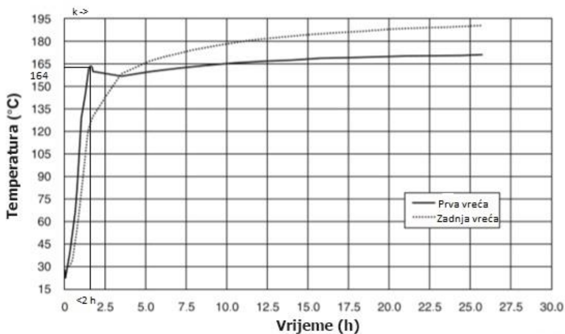
Slika 6-3. Promjena temperature cementne kaše s vremenom (North i dr., 2000).
