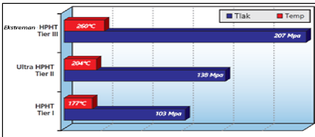
Slika 2-2. Prikaz klasifikacije HPHT uvjeta koju koristi kompanija Baker Hughes (Shadravan i Amani, 2012)
