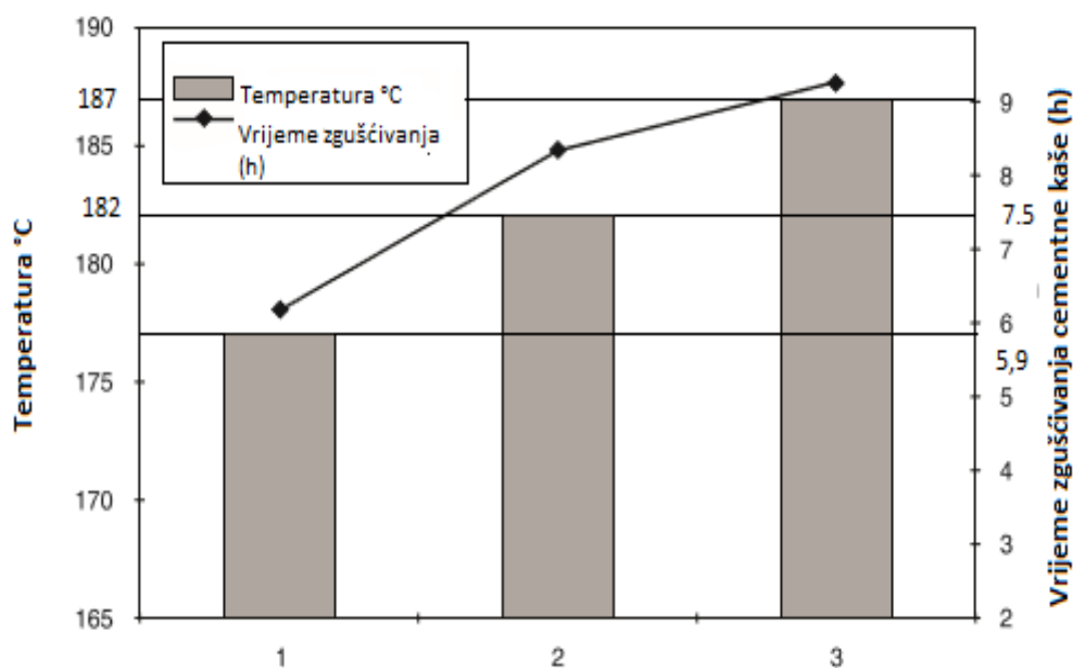
Slika 6-6. Osjetljivost cementne kaše na promjenu temperature i koncentraciju usporivača na 182 °C (North i dr., 2000)
