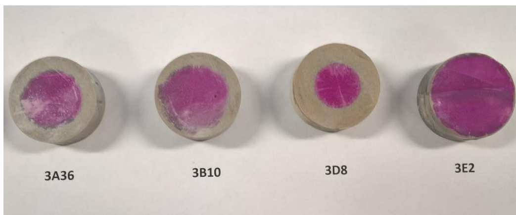
Slika 4-31. Uzorci cementnog kamena premazani fenolftaleinom nakon izlaganja vodi zasićenoj s CO 2
