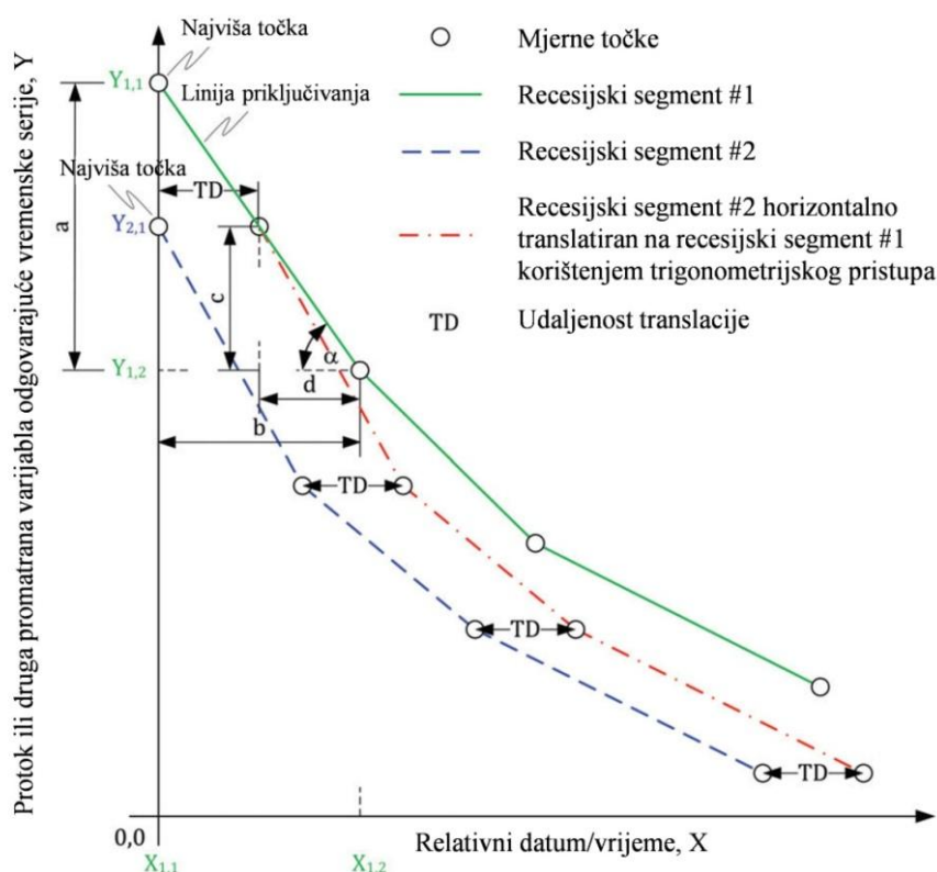
Slika 6.2. Koncept korištenja trigonometrijskih funkcija prilikom translacije recesijskih segmenata (Posavec i dr., 2017.)
