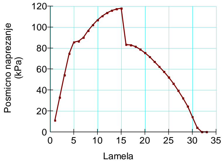
Slika 5-12 Posmično naprezanje duž klizne plohe
