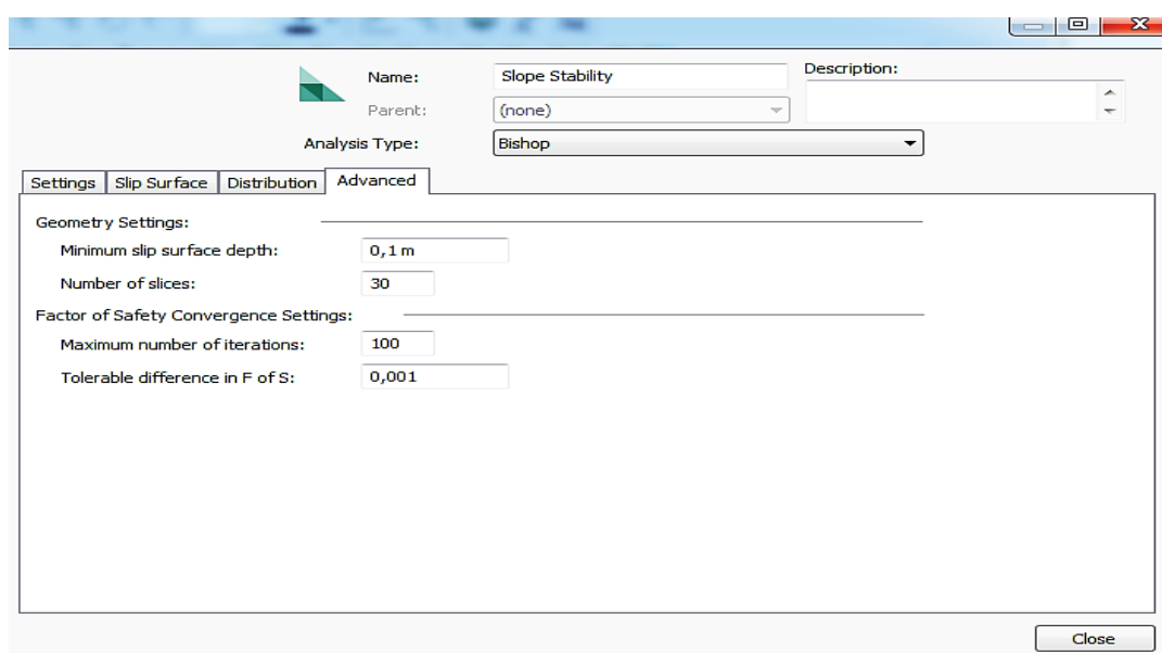
Slika 4-1 Ulazni parametri Bishopove metode
