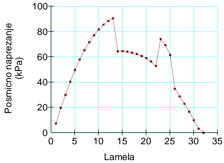
Slika 5-16 Posmčno naprežanje duž klizne plohe
