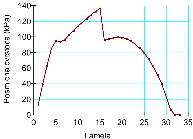
Slika 6-11 Posmična čvrstoća duž klizne plohe dobivena MP metodom
