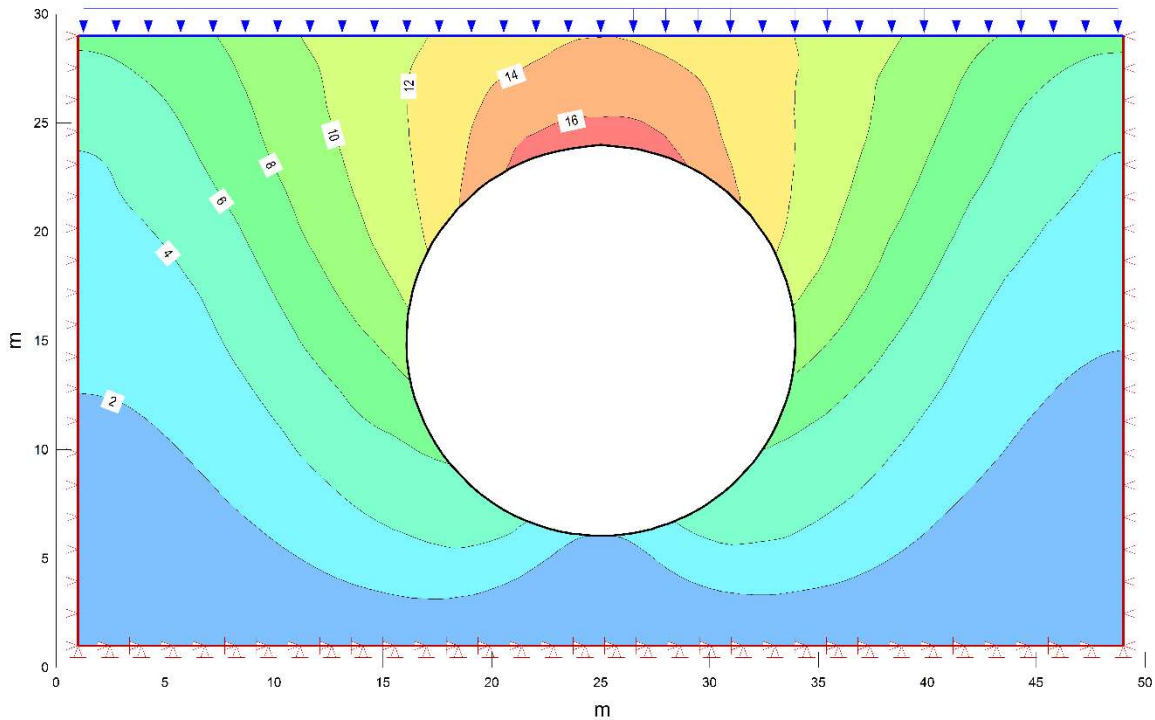
Slika 4-37 Pomaci u fazi iskopa tunela (iznosi u mm).
