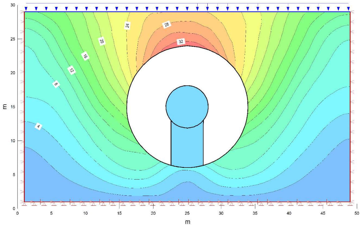
Slika 4-38 Pomaci u fazi ugradnje spremnika (iznosi u mm).
