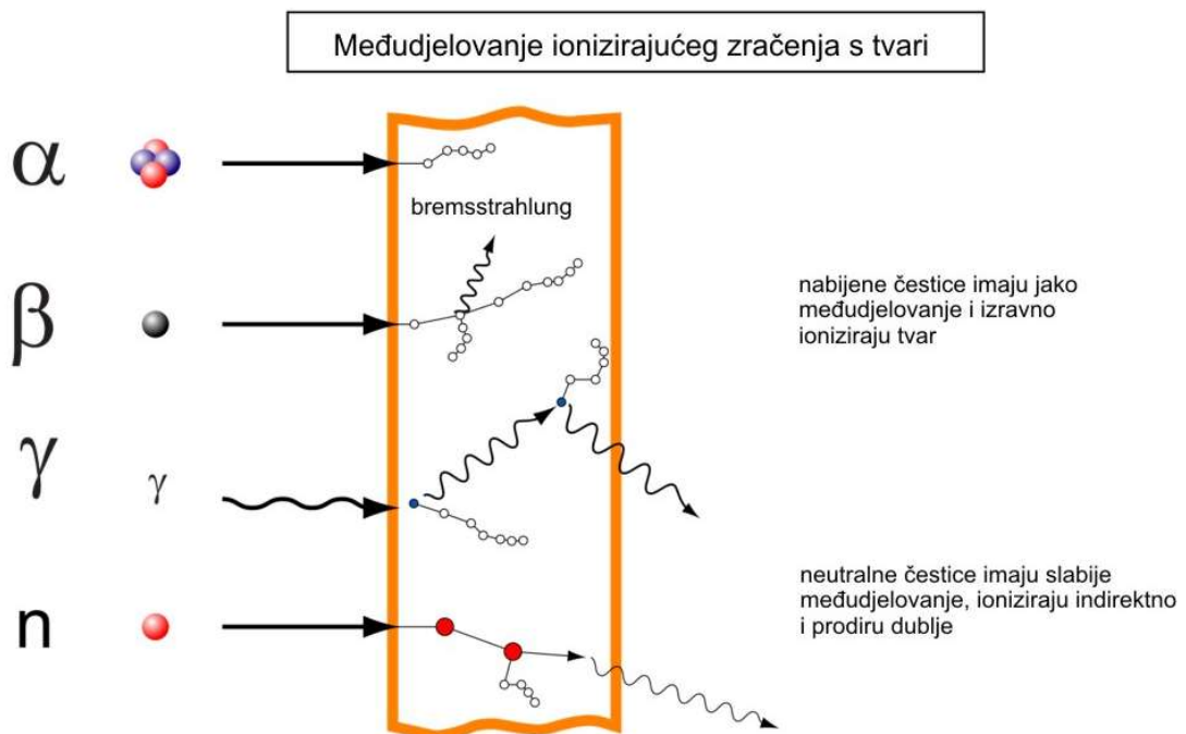
Slika 2-9 Grafički prikaz međudjelovanja ionizirajućeg zračenja s tvarima (NAPYIKENOBI, 2019)
