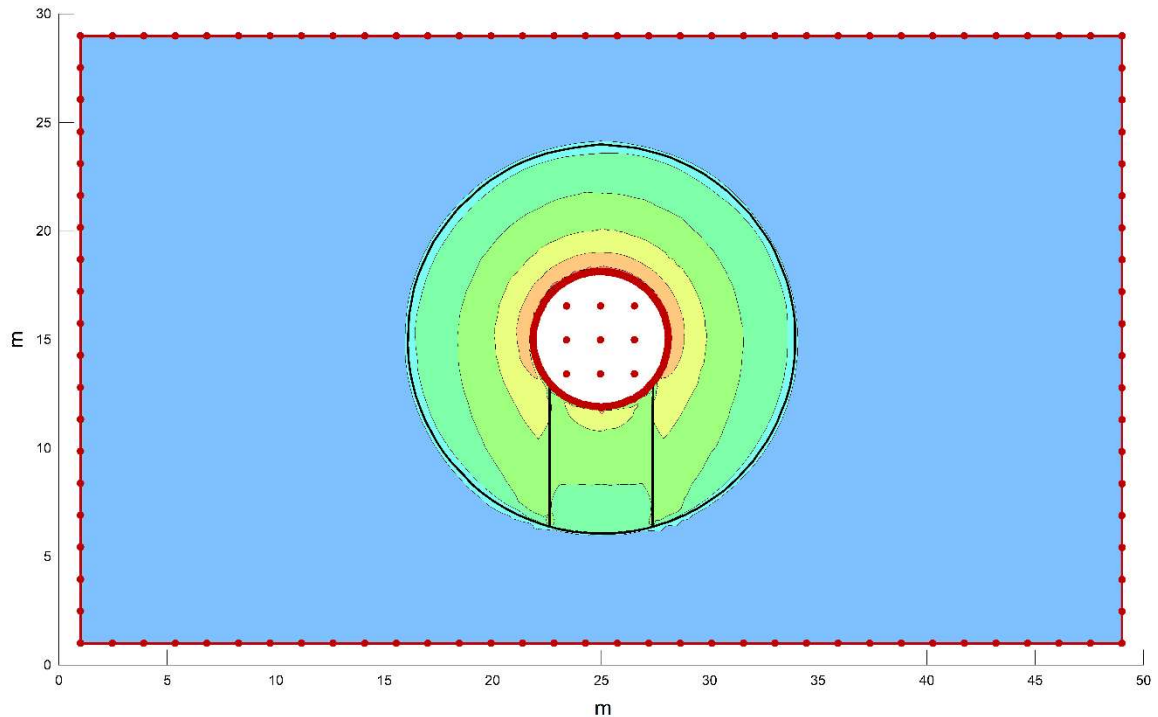
Slika 4-48 Model širenja topline – gradijent topline (x i y smjer) kroz bentonit i stijenu.
