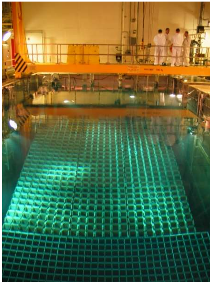
Slika 2-23 Bazen za istrošeno gorivo (ZBRINJAVANJE RAO, 2019)
