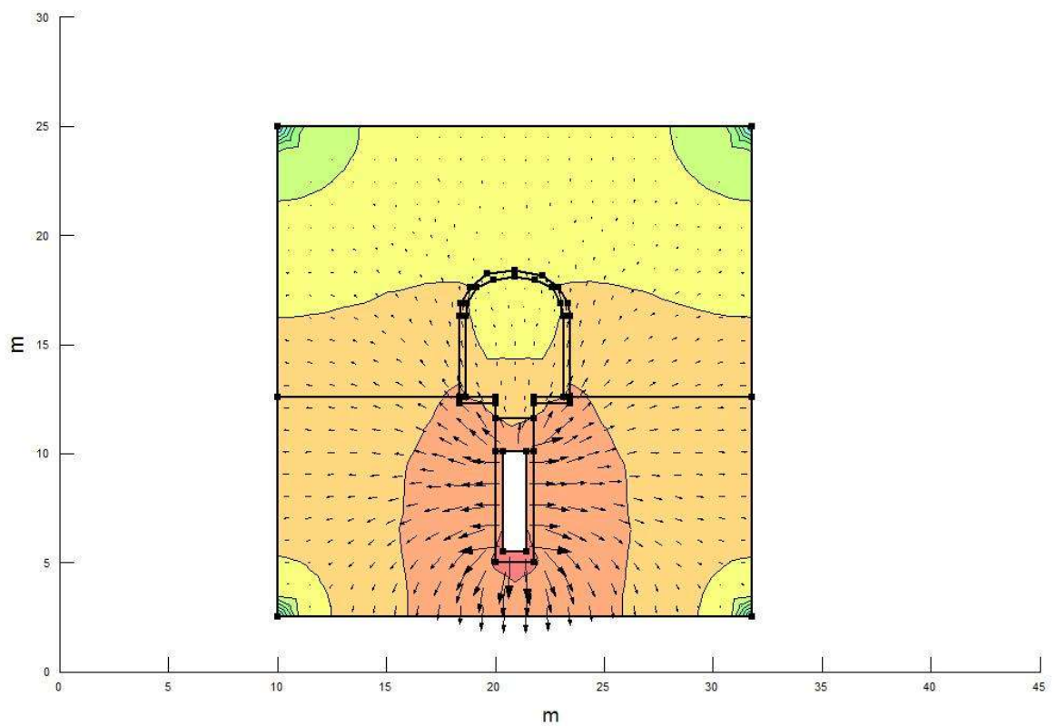
Slika 4-27 Model širenja topline – toplinski tok (x i y smjer) kroz stijenu.
