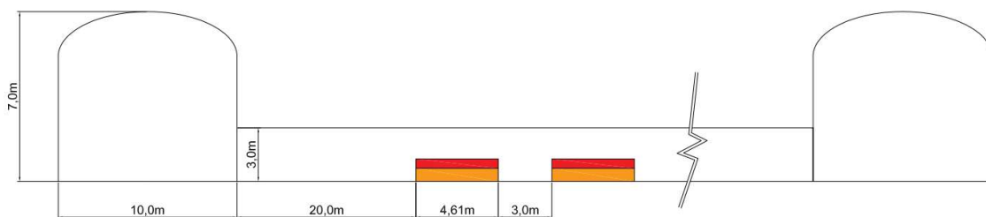
Slika 3-12 Prikaz rasporeda spremnika u odlagališnom tunelu za Koncept-4 (prema: NAGRA, 2009 i 2002)
